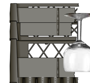
2 Extender 165 mm / 159 mm # GR-9-P3-BLK # GR-16-P3-BLK # GR-49-P3-BLK
